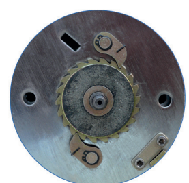
Dubbele rempal
